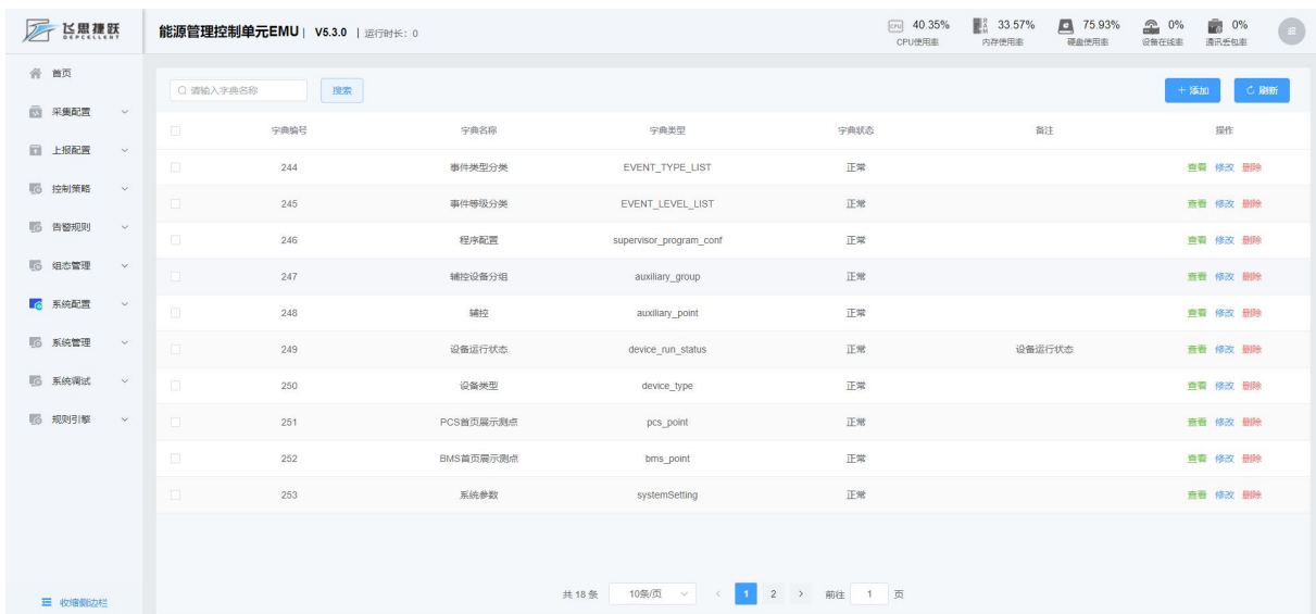
图 4-26 字典管理
