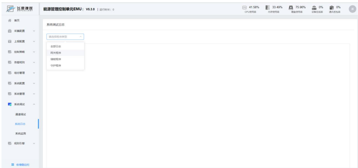
图 4-32 系统日志
