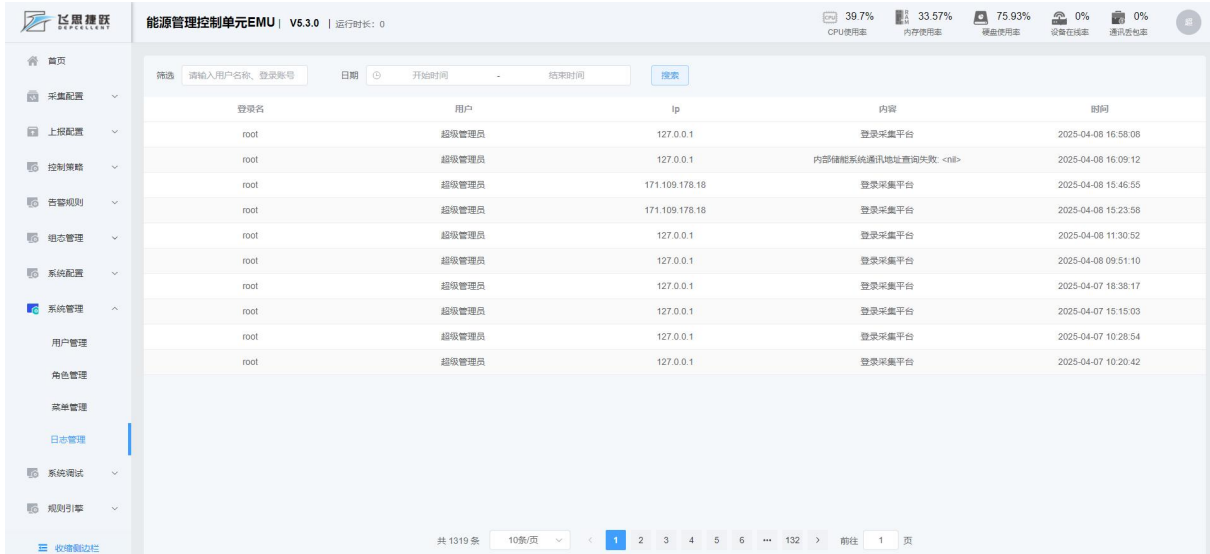
图 4-30 日志管理
