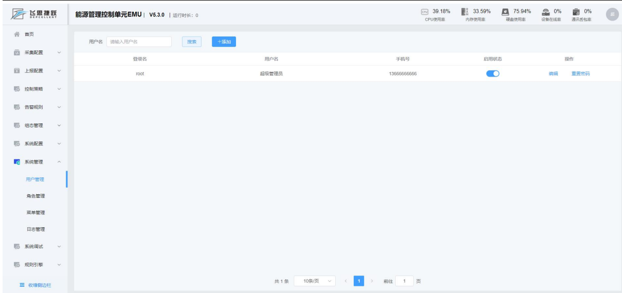
图 4-27 用户管理
