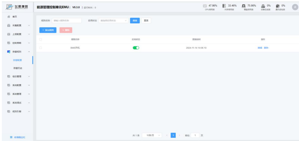
图 4-20 告警配置
