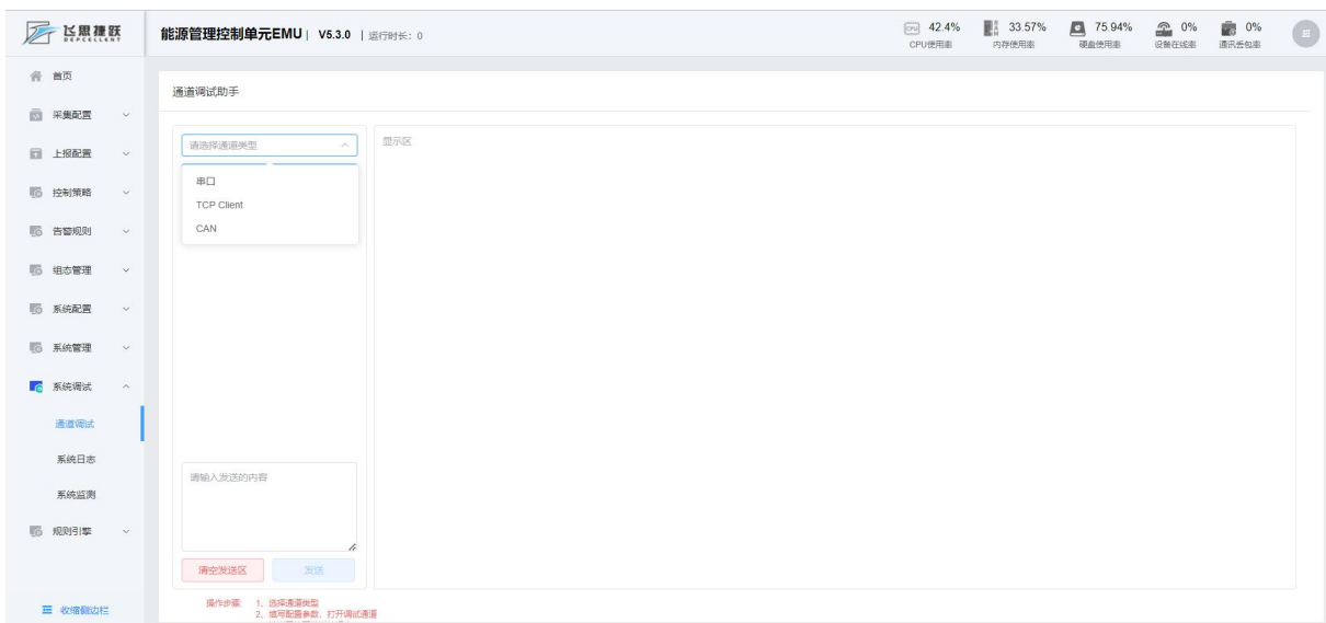
图 4-31 通道调试
