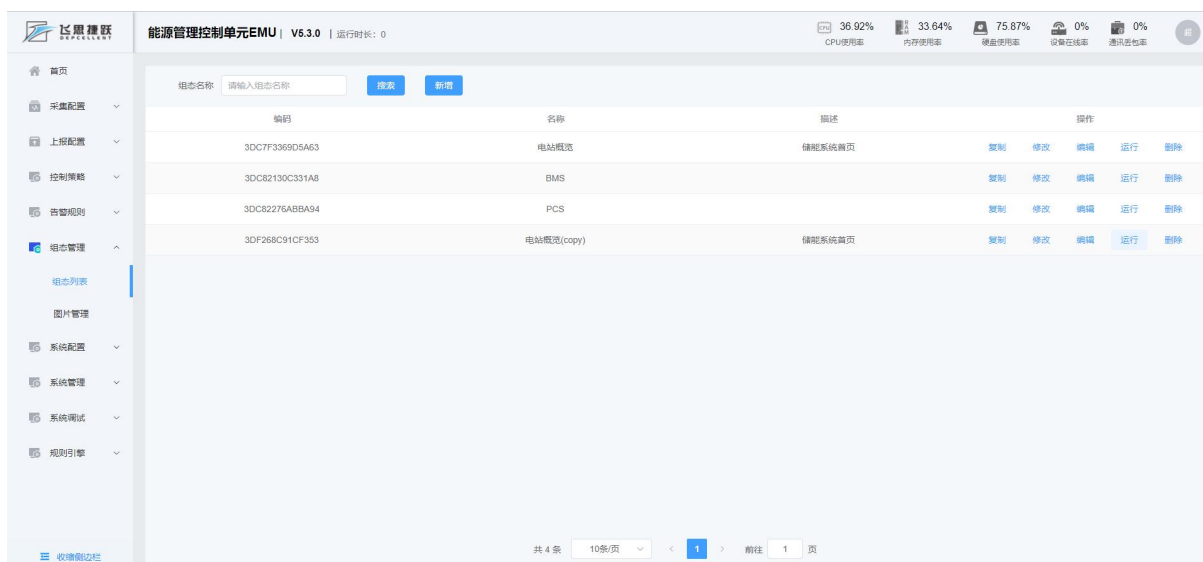
图 4-22 组态管理
