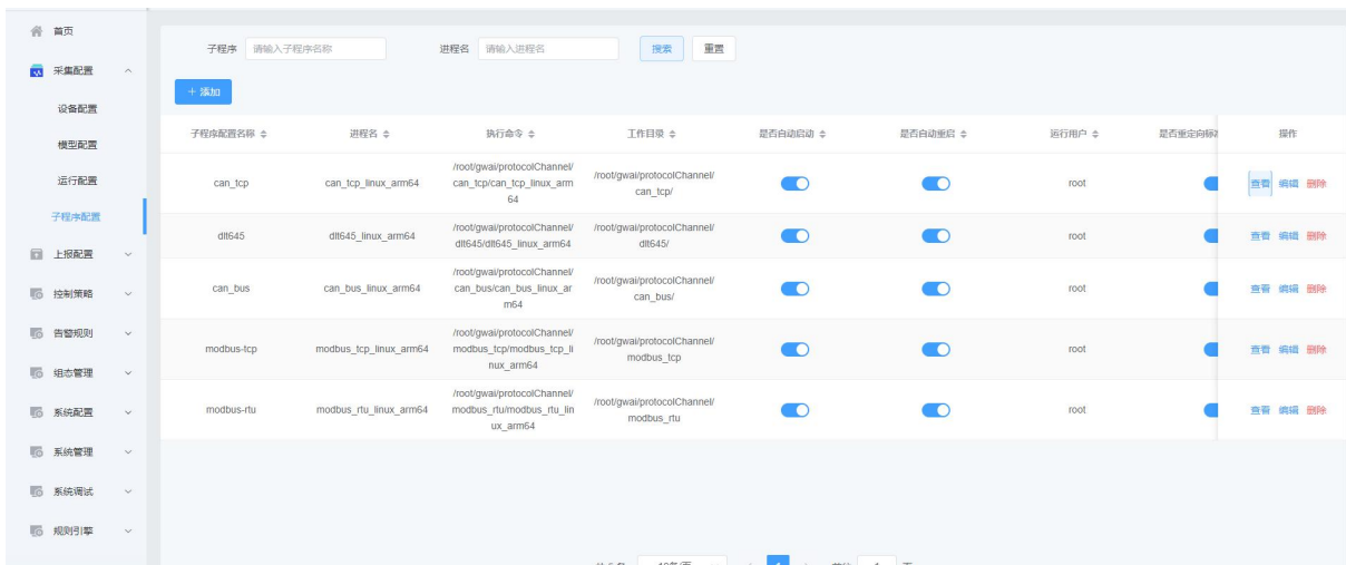
图 4-17 子程序配置
