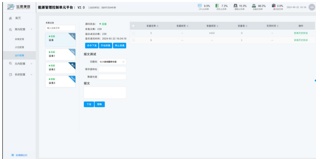
图 4-15 调试
