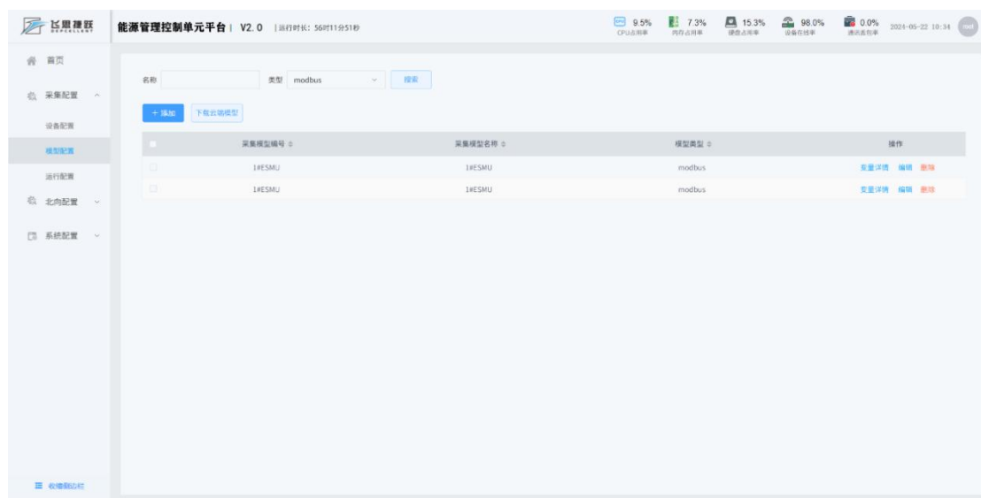
图 4-12 模型配置
