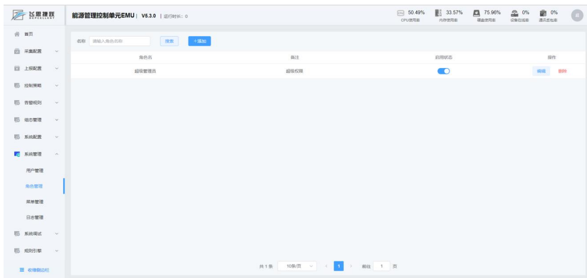
图 4-28 角色管理
