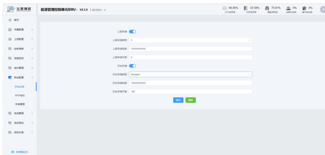
图 4-24 存储设置
