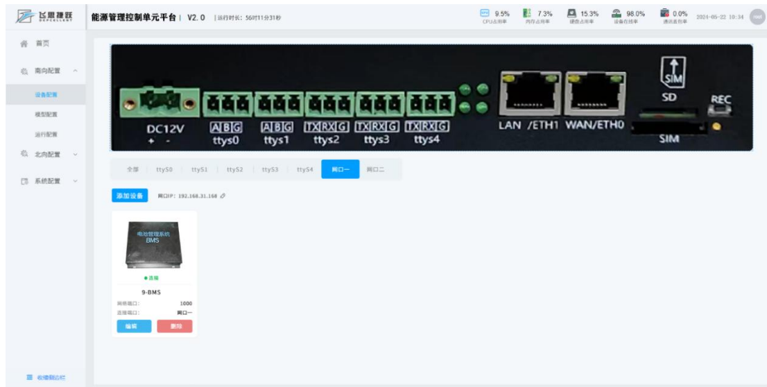
图 4-8 网口设备
