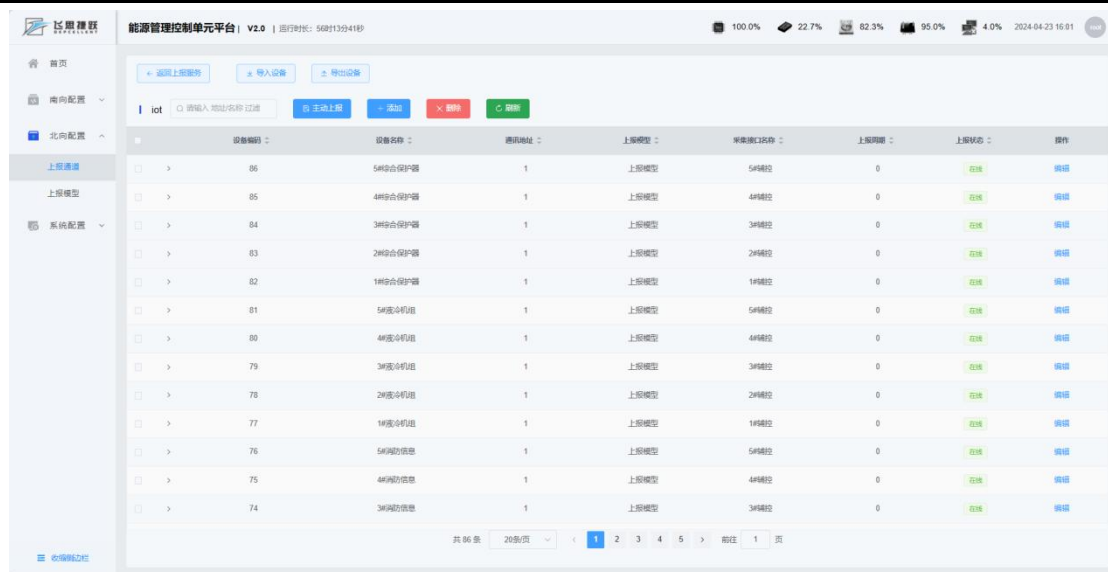
图 4-19 上报节点
