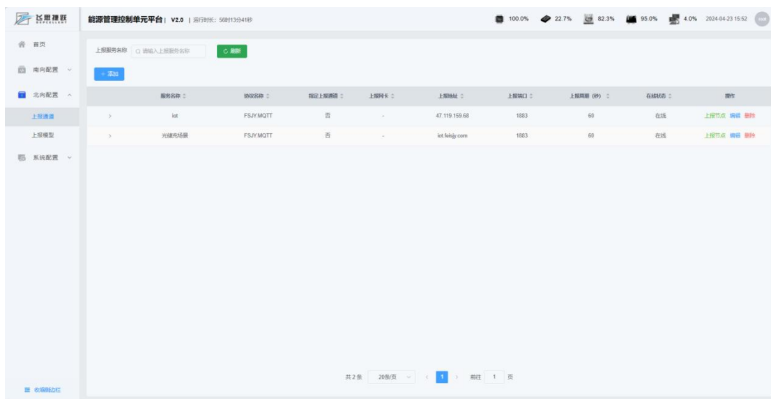
图 4-18 上报通道
