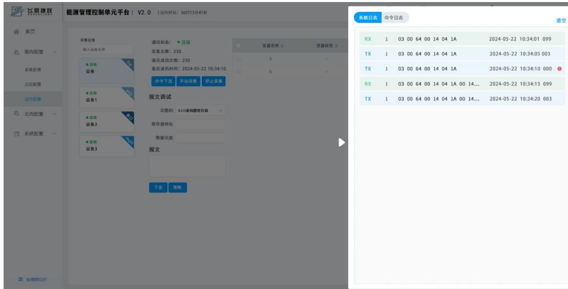
图 4-16 系统日志
