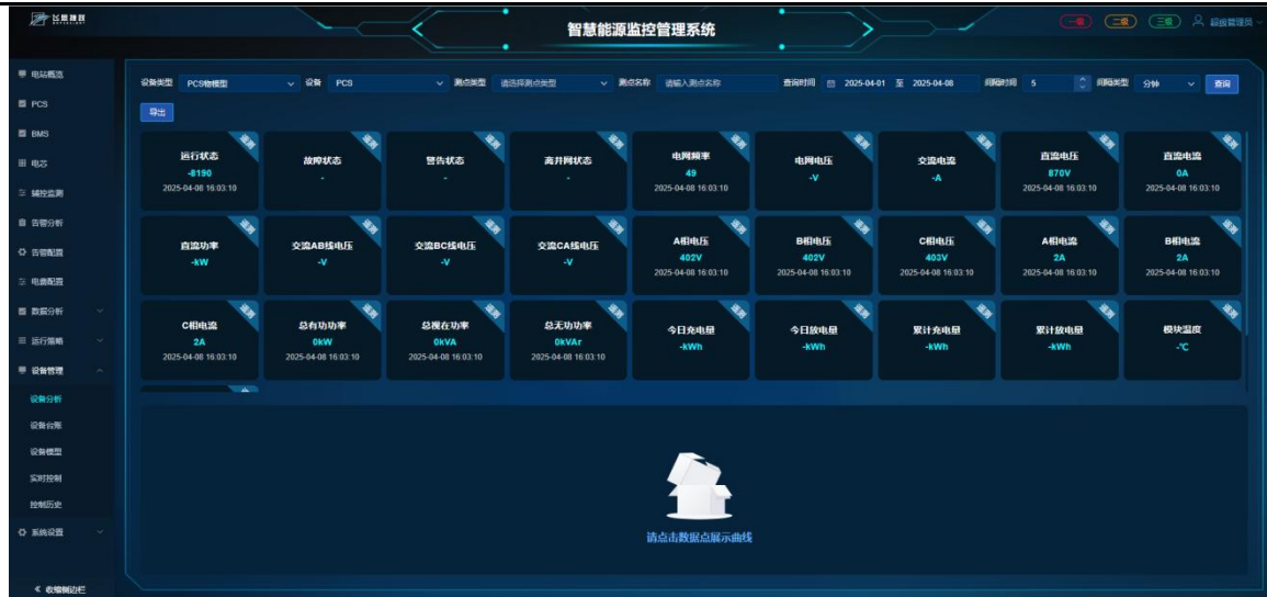
图 3-18 设备分析
