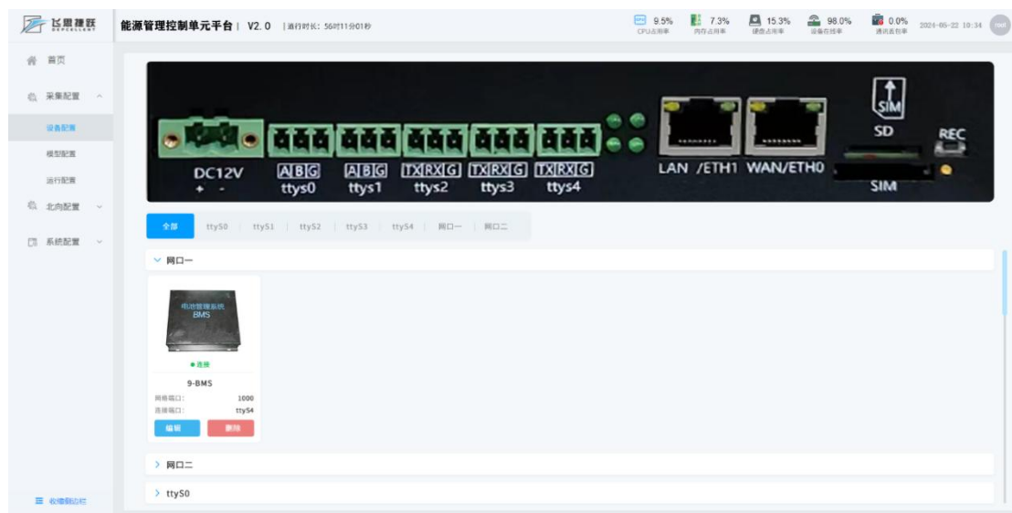
图 4-3 全部设备
