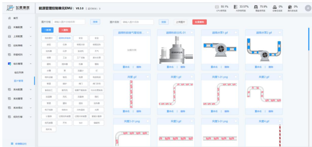
图 4-23 图片管理
