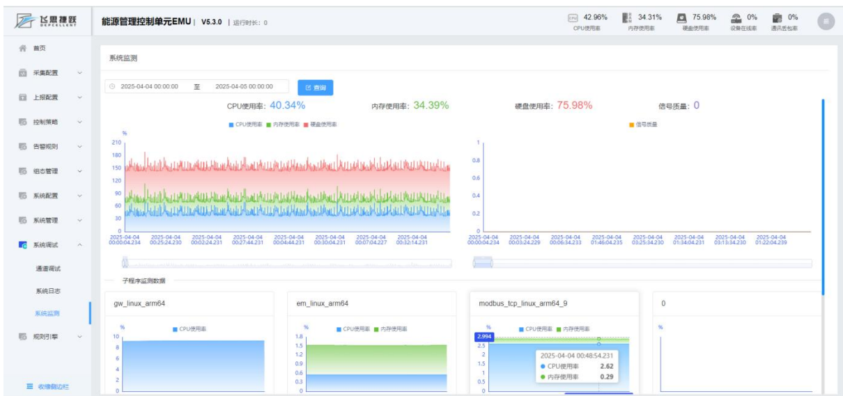
图 4-33 系统监测
